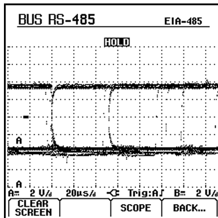
Рис. 3. Новые изображения экрана параметров состояния шины (слева) и глазковой диаграммы (справа), полученные после замены кабеля и прокладки его вдали от линии питания. Ясно видно улучшение работы сети, все параметры соответствуют требованиям
