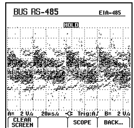
Рис. 2. Слева: показания уровня напряжения сигнала, джиттера и выброса на фронте импульса выходили за пределы допустимых значений для данной шины. Справа: альтернативное представление сигналов шины при помощи глазковой диаграммы отображает искажение сигнала в данной зоне, что свидетельствует о наличии в шине высокого уровня помех
